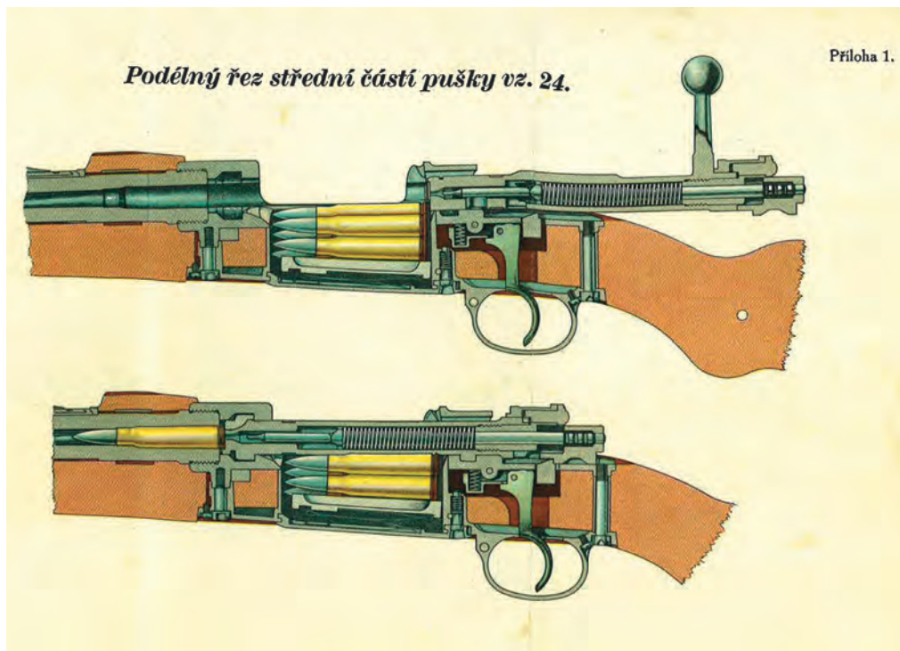
Částečný řez puškou vzor 24. (Rezina)
