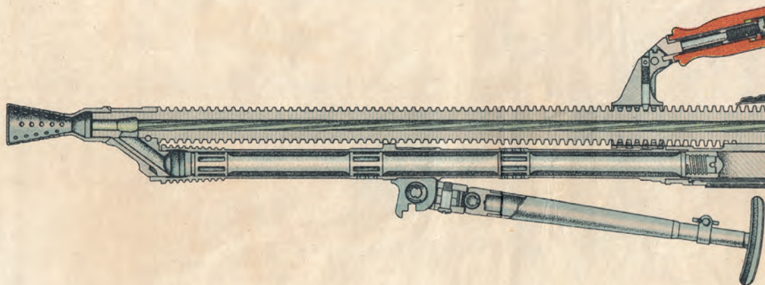
Podélný řez kulometem vz. 26.
