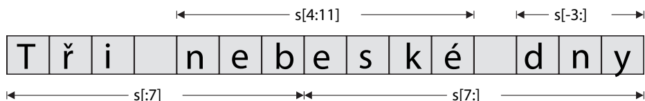
Obrázek 2.2: Řezání posloupnosti
