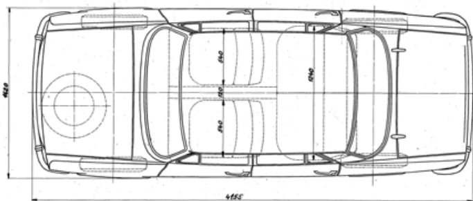
Výkres prototypu sedanu Š 717 s novou kabinou datovaný 5. května 1965
