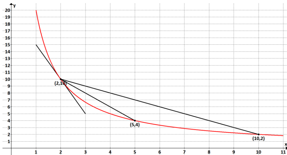
Obrázek 1.3 Mocninná funkce
