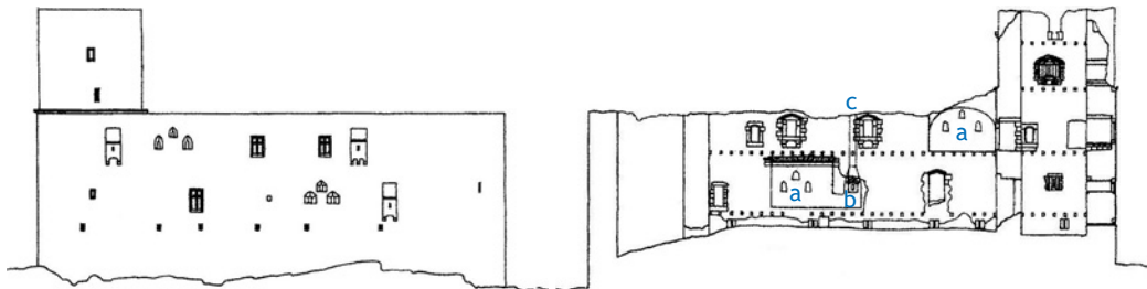
1.06 Roubené komory na hradě Radyni (exteriér, interiér): a – roubená komora, b – krb, c – komin [148 Menclová]
