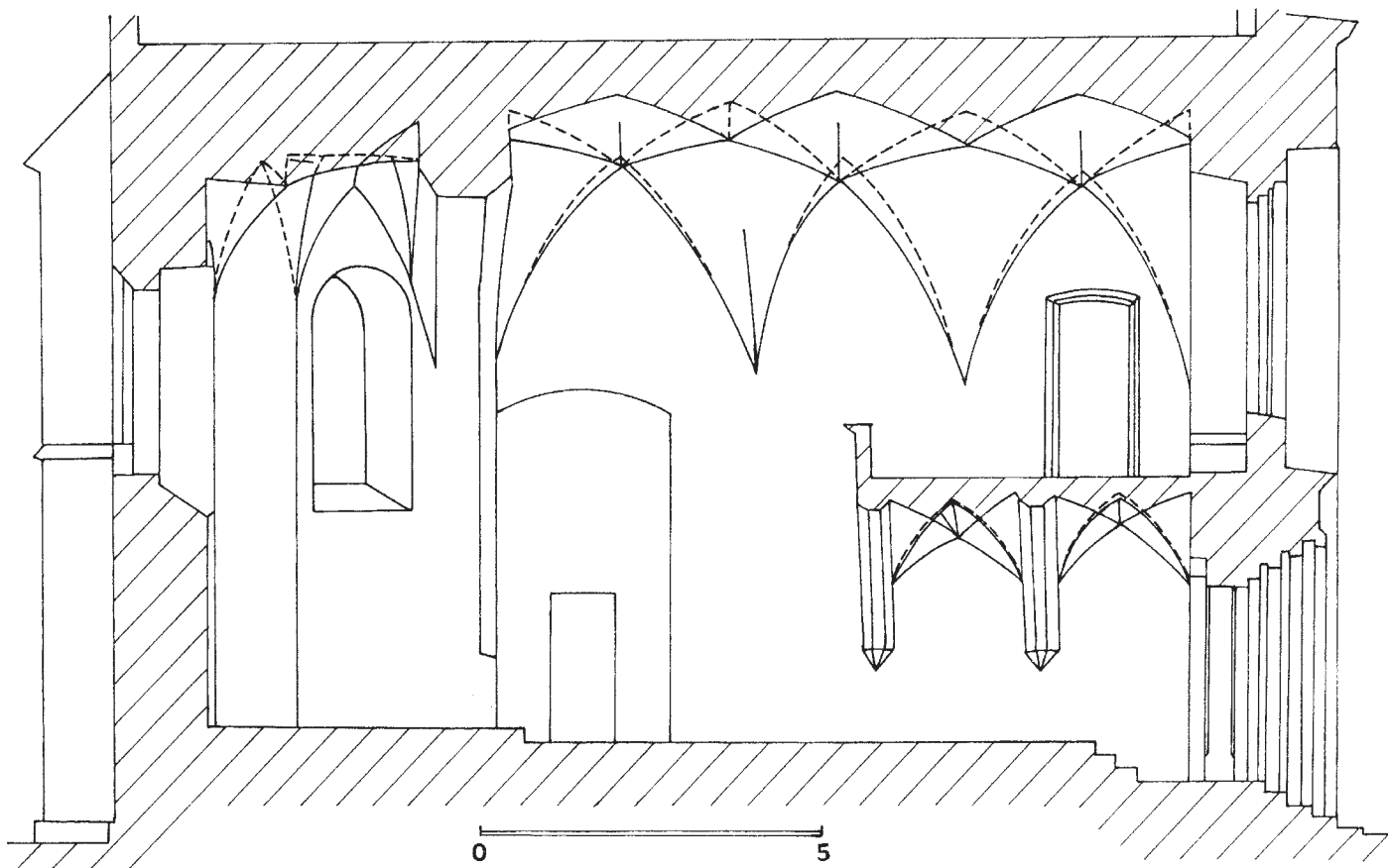
Obr. 8. Bor u Tachova. Podélný řez hradní kaplí (podle M. a O. Radových)
