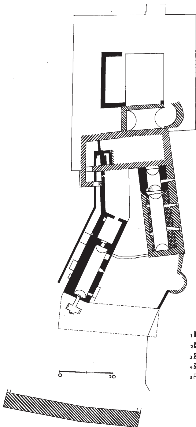
Obr. 2. Bechyně. Půdorys suterénu jádra (podklad podle J. Muka, doplněno, upraveno). 1 – starší gotické zdivo, 2 – pravděpodobně starší gotické zdivo, 3 – mladší gotické zdivo, 4 – pozdně gotické zdivo, 5 – zadní zbořený palác podle plánu z roku 1764
