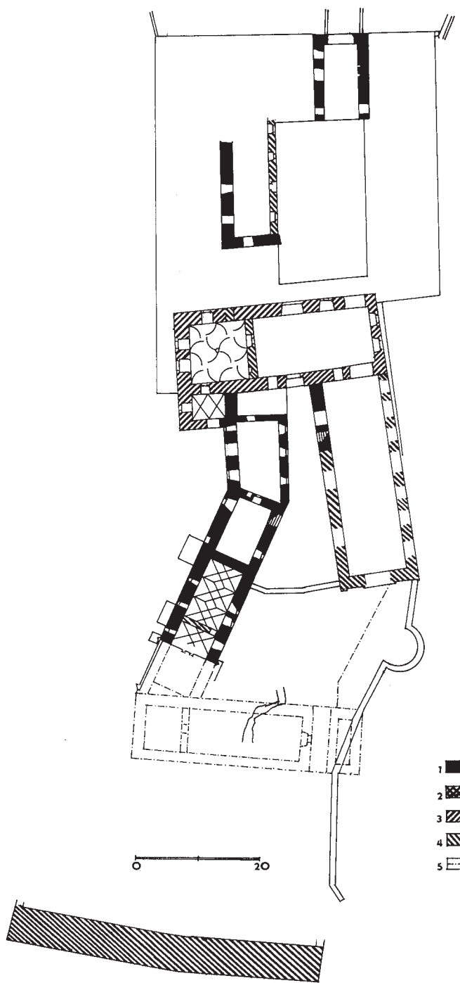
Obr. 3. Bechyně. Půdorys přízemí jádra (podklad podle J. Muka, doplněno, upraveno). 1 – starší gotické zdivo, 2 – pravděpodobně starší gotické zdivo, 3 – mladší gotické zdivo, 4 – pozdně gotické zdivo, 5 – zadní zbořený palác podle plánu z roku 1764
