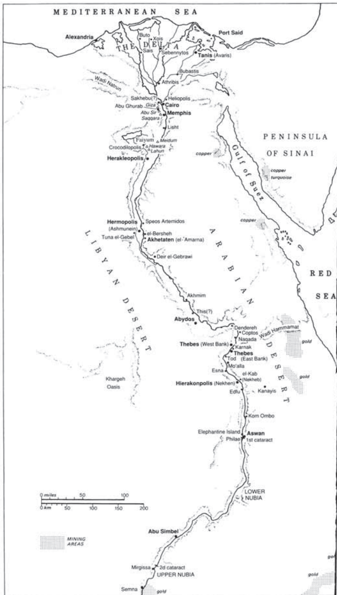
Egypt. Údolí Nilu a delta ukazující místa zmíněná v textu. Nakreslili Brian a Connie Dearovi. Přetištěno z Jonh Ruffle, The Egyptians (1977), str. 12, se svolením Phaidon Press, Oxford.
