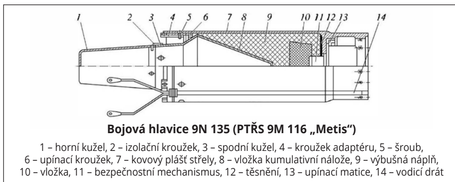
Obr. 1-2: Kumulativní hlavice. (Zdroj: A. P. Orlov, Osnovy ustrojenstva i funkcionirovanija snarjadov RSZO , upraveno autorem)
