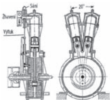
▲ Obr. 2.8 Motor Daimler V2
