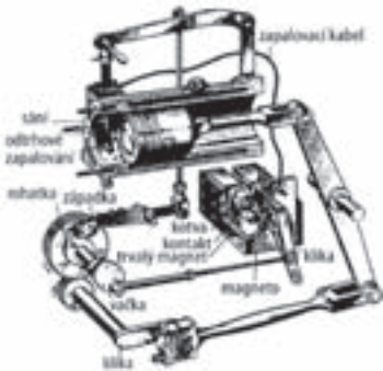
▲ Obr. 2.13 Vůz Marcus s benzínovým motorem a detail motoru
