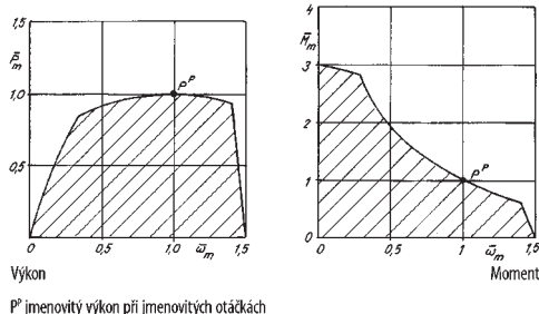
▲ Obr. 1.12 Bezrozměrná charakteristika parního stroje
