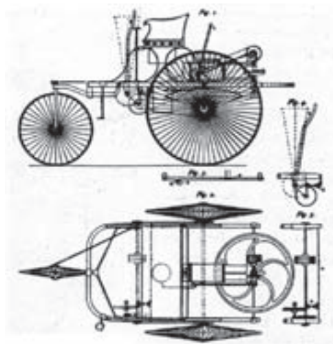
▲ Obr. 2.10 Vůz Benz podle náčrtu v patentové dokumentaci
